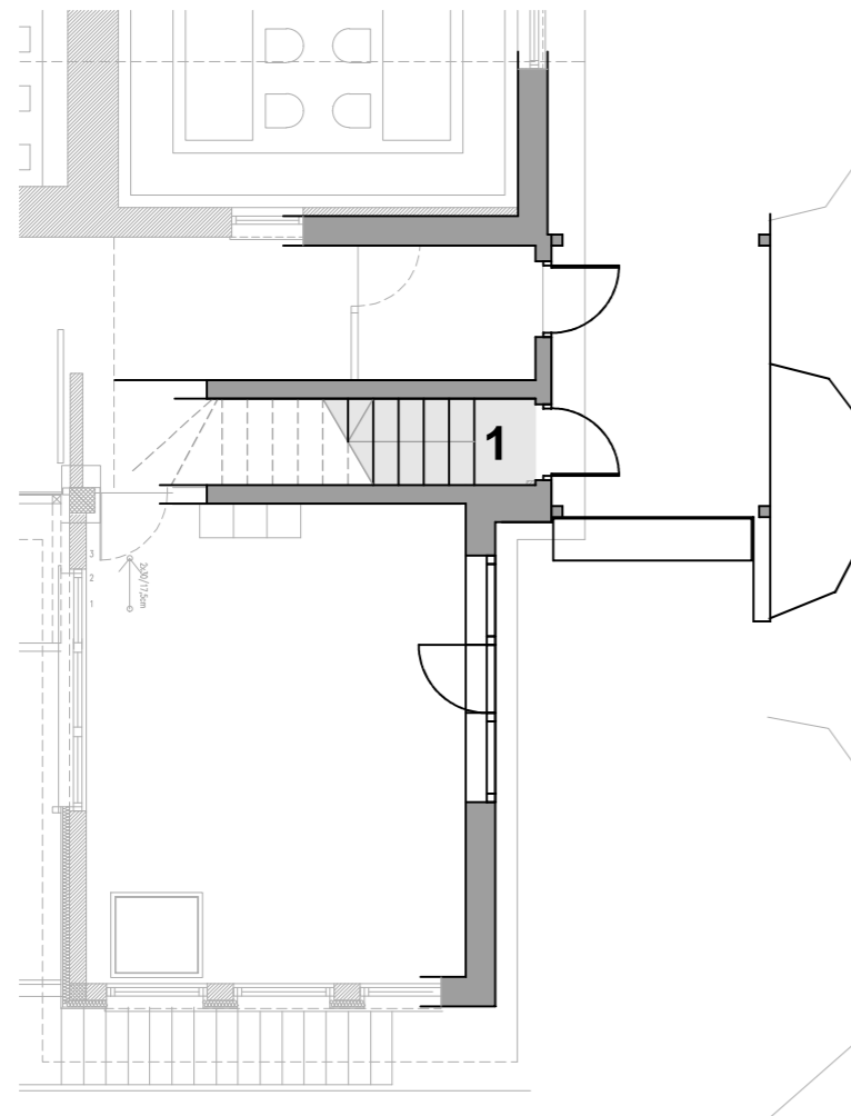
Pritičje M 1:100
