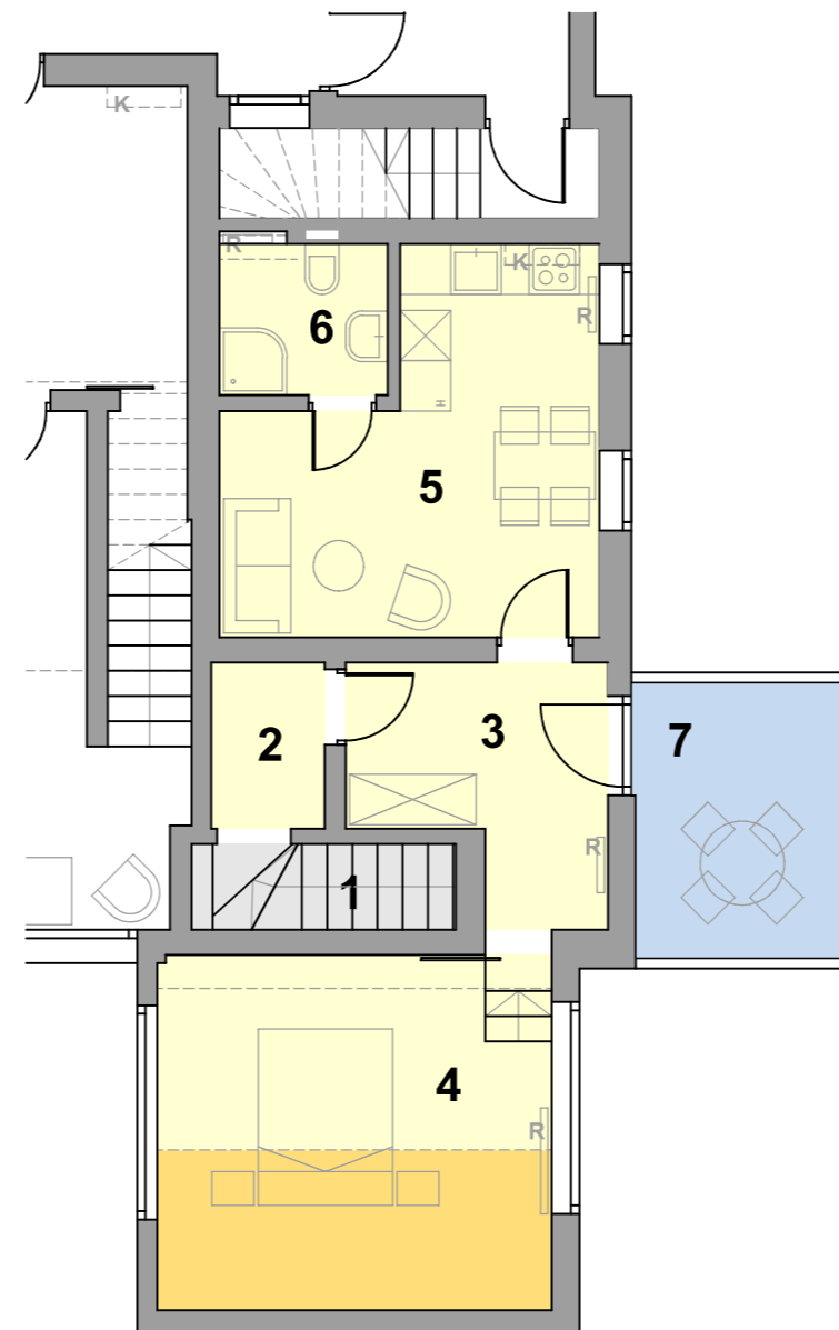
1. nadstropje M 1:100
