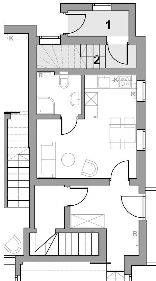
1. nadstropje M 1:100
