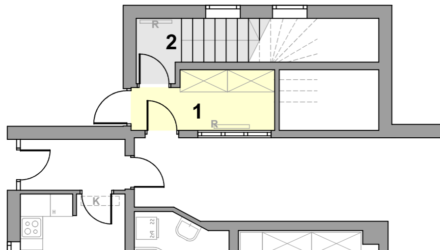
1. nadstropje M 1:100
