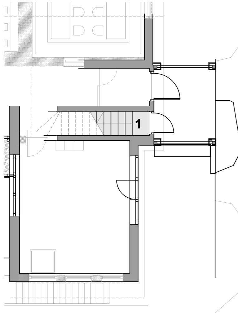
Pritličje M 1:100
