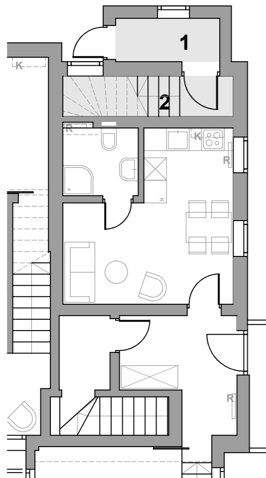
1. nadstropje M 1:100
