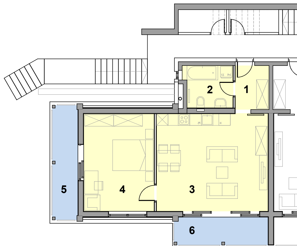
1. nadstropje M 1:100
